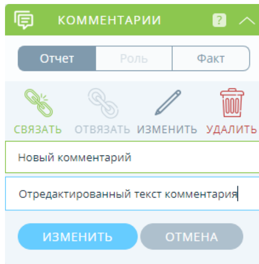
Рисунок 40 - Редактирование комментария.
