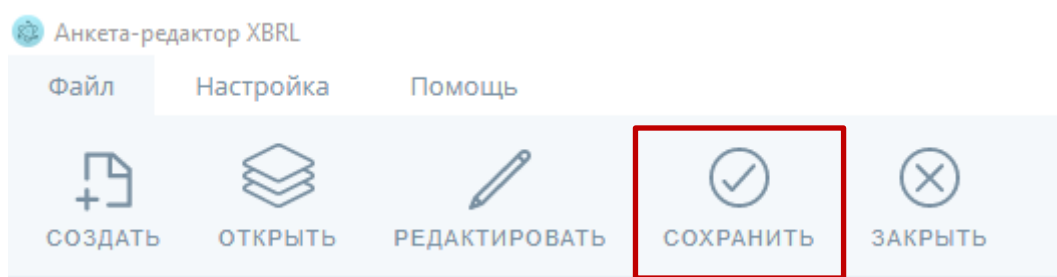
Рисунок 5 – кнопка «Сохранить».
